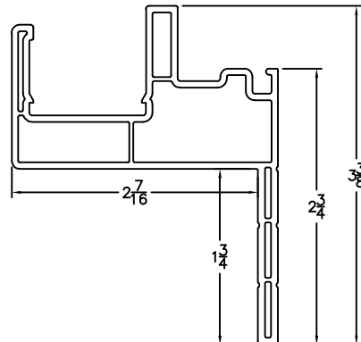
STUCCO Frame
