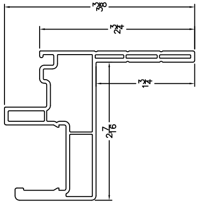
STUCCO Frame
